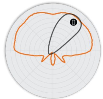
Abbildung 5. T310d 5 GHz-Elevation-Antennenmuster
