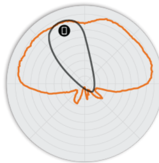
Abbildung 4. T310d 2,4 GHz-Elevation-Antennenmuster
