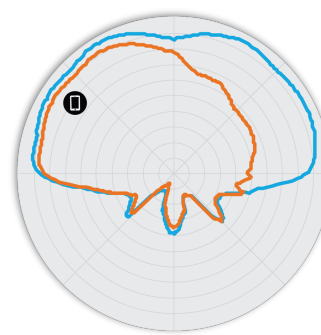
图 5. R850 5GHz 俯仰 天线模式
