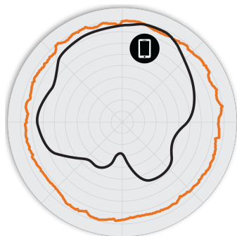
図 2. R850 2.4GHz アジマス アンテナ パターン
