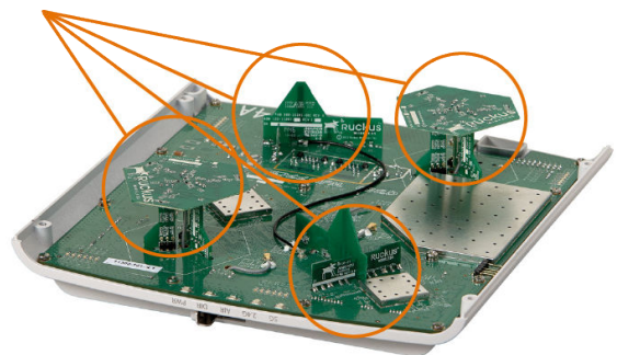
BeamFlex+ 적응형 안테나 기술
