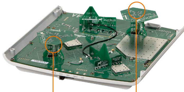
BeamFlex+ 적응형 안테나 기술
