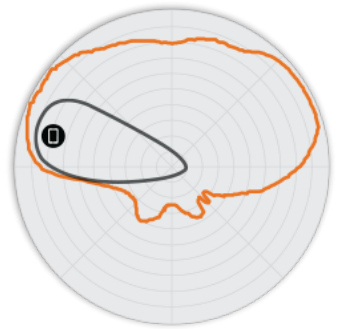
FIGURE 5 Diagrammes d'antennes Élévation R610 5 GHz
