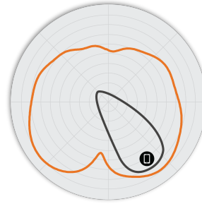
Figura 4. R350 2,4 GHz: patrones de antena en elevación
