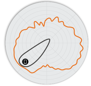
Figura 5. R350 5 GHz: patrones de antena en elevación
