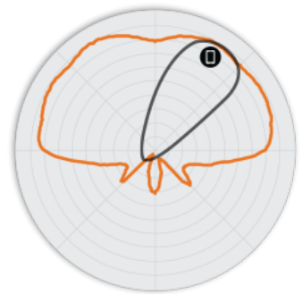
圖 5 R310 5GHz 仰角天線模式
