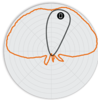
圖 4 R310 2.4GHz 仰角天線模式
