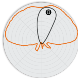
図 4. R310 2.4GHz エレベーション アンテナ パターン
