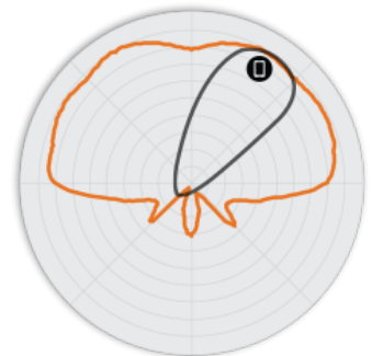
図 5. R310 5GHz エレベーション アンテナ パターン
