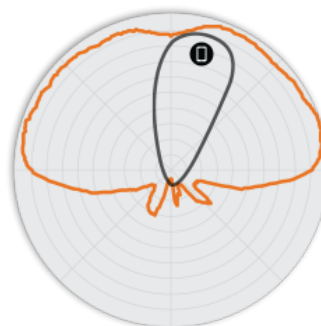
Figure 4. R310 2,4 GHz: patrones de antena en elevación
