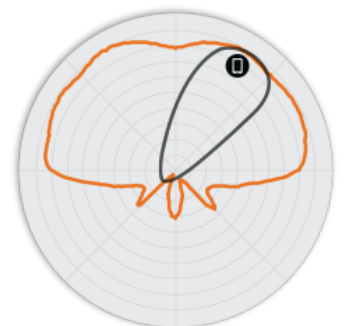
Figure 5. R310 5GHz: patrones de antena en elevación
